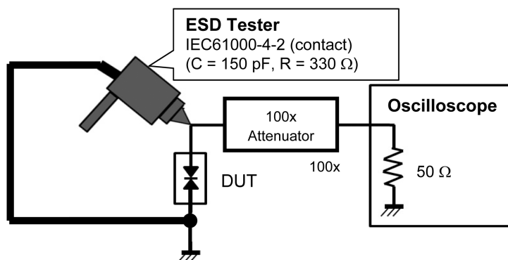
Fig. 6.1.5 IEC61000-4-2 (Contact)
