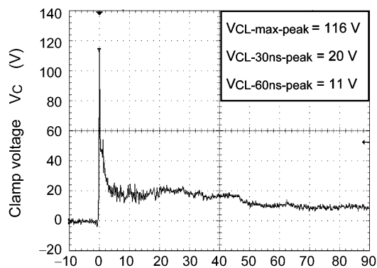
Fig. 6.1.1 +8 kV
