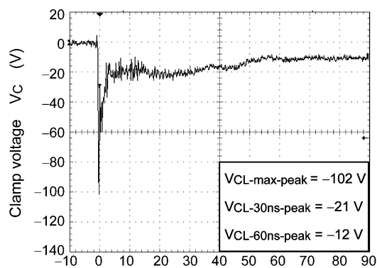
Fig. 6.1.2 -8 kV
