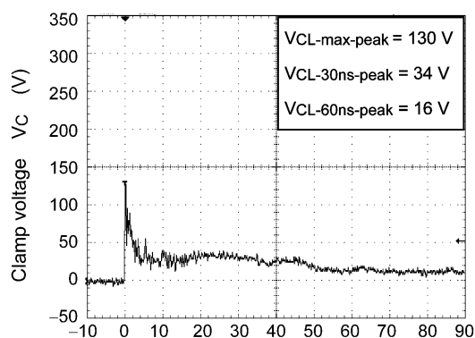
Fig. 6.1.3 +15 kV
