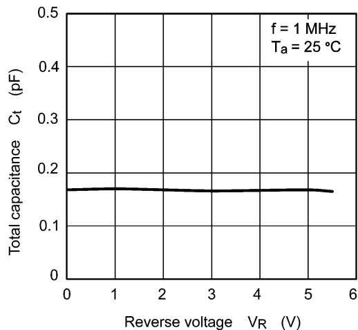
Fig. 9.3 C_t - V_R
