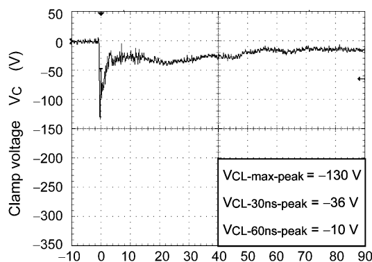
Fig. 6.1.4 -15 kV
